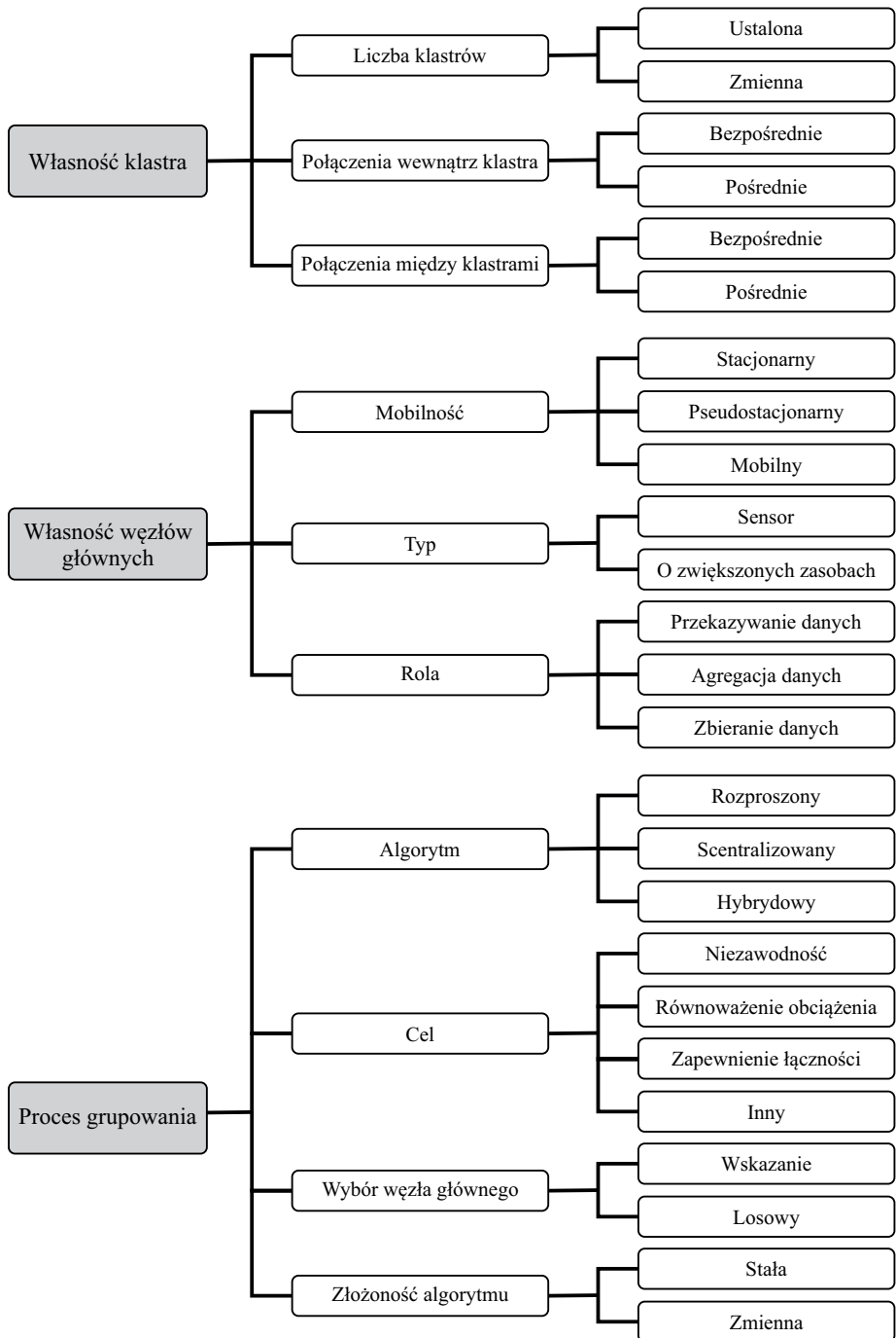
Rysunek 10.1. Taksonomia algorytmów grupowania
