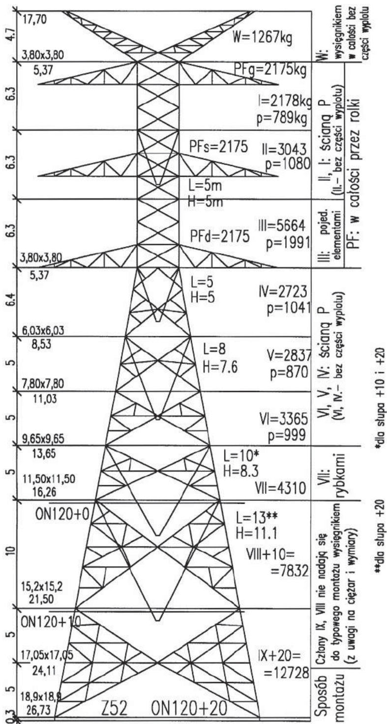
Rys. 13.120. Montaż wysokościowy słupa Z52 ON120+20 według [2.51]
